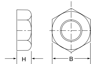
Nut
